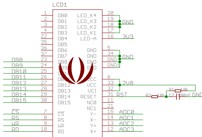
2.8" ST7781R 8bit LCD
